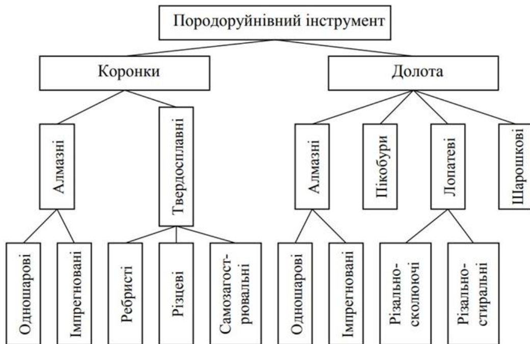
Рис. 5.1 – Схема класифікації породоруйнівного інструмента
