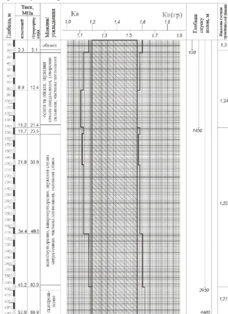
Рисунок 3.1 – Суміщений графік зміни тисків
