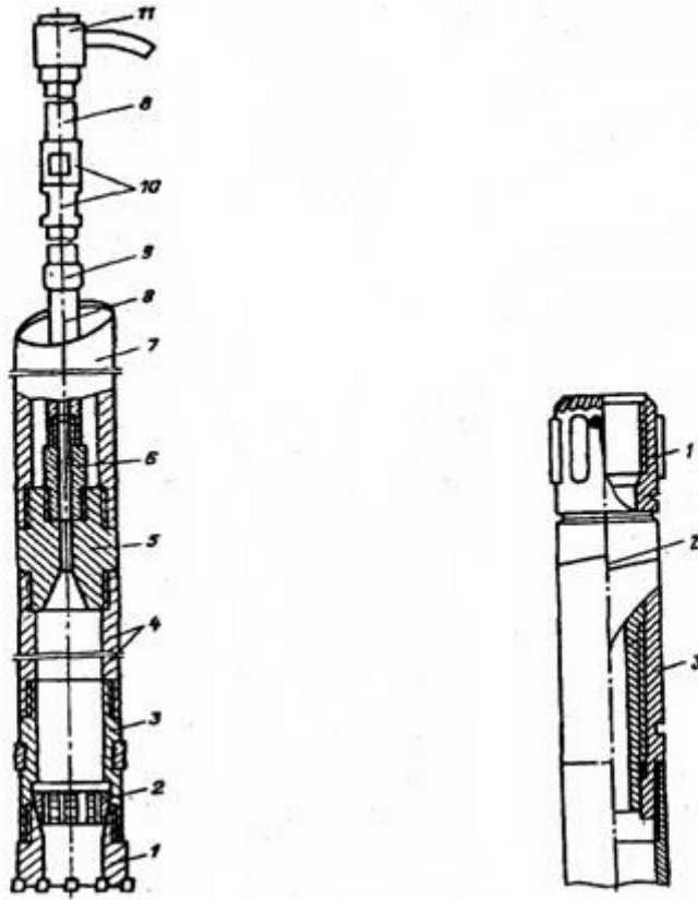
Рис. 5.2. – Буровий снаряд: колонковий набір:
