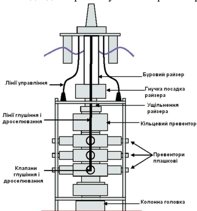
Рис. 7.1. Схема конструкції верхньої частини свердловини з підводним противикидним обладнанням
