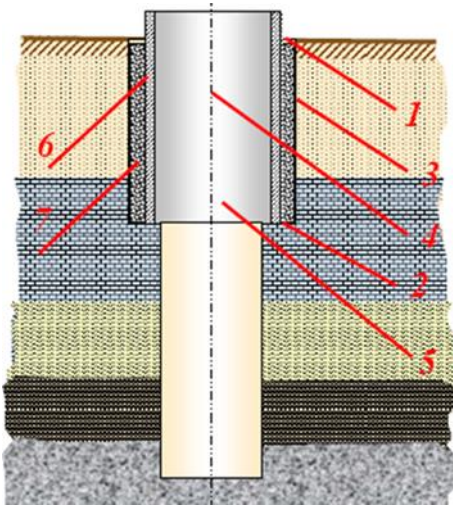
Рис. 2.1. – Основні елементи бурової свердловини
